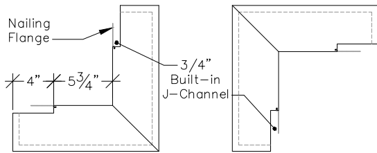
Top 1"=1'-0"
